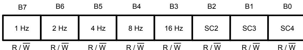
图14 INT1寄存器 (频率设定数据)
