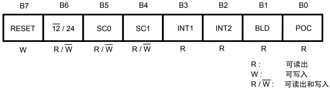
图11 状态寄存器1
