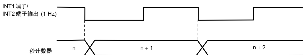
图17 1 Hz的时钟输出和秒计数器
