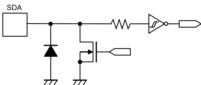
图4 SDA端子
