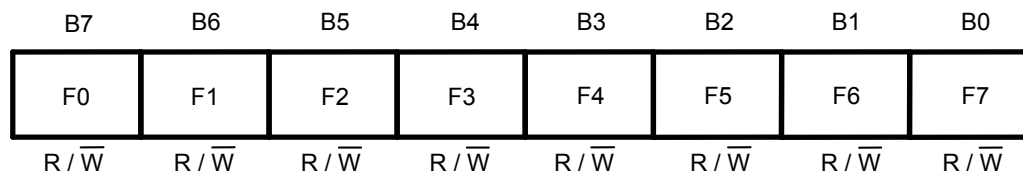
图19 自由寄存器
