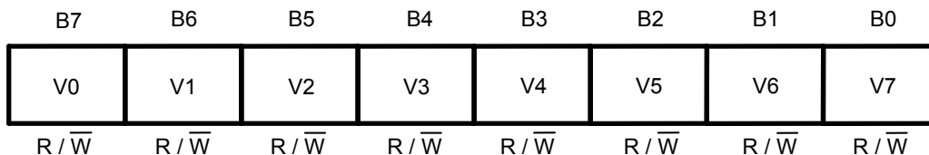
图18 时钟校正寄存器
