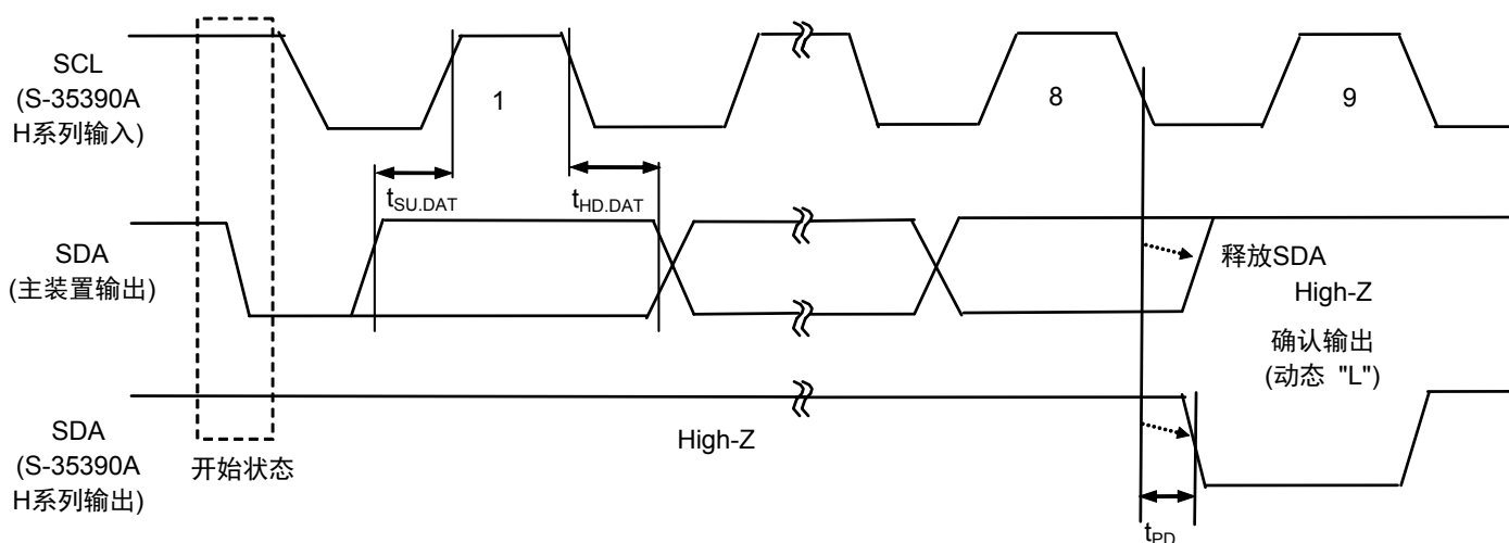
图33 确认输出时序
