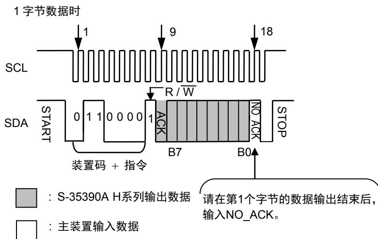
图34 数据读出例1 (1字节数据寄存器)
