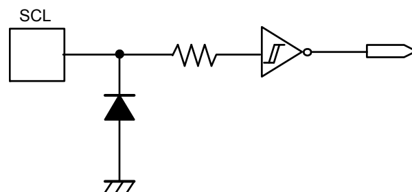
图5 SCL端子
