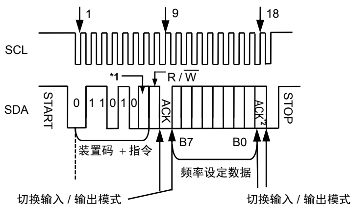
图41 INT1寄存器存取、INT2寄存器存取
