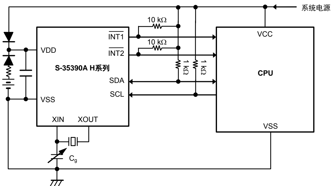
图48 应用电路2
