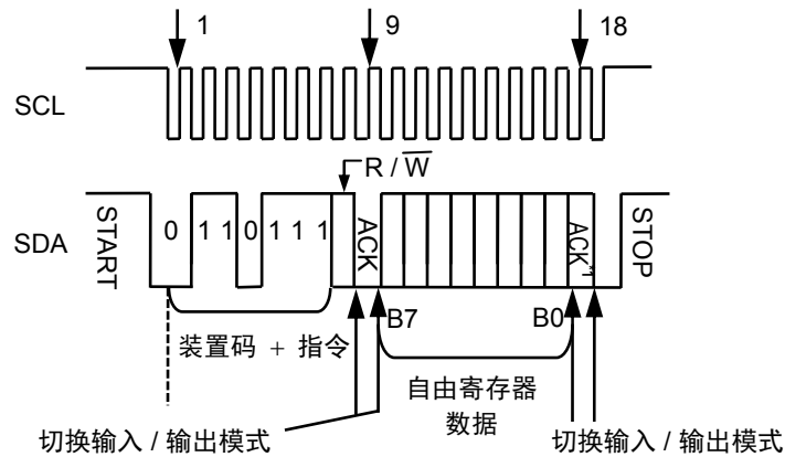
图44 自由寄存器存取
