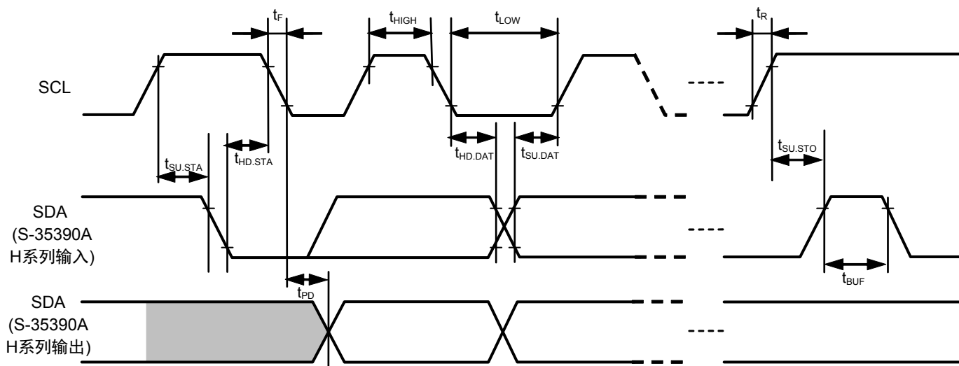
图8 总线时序
