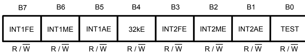
图12 状态寄存器2
