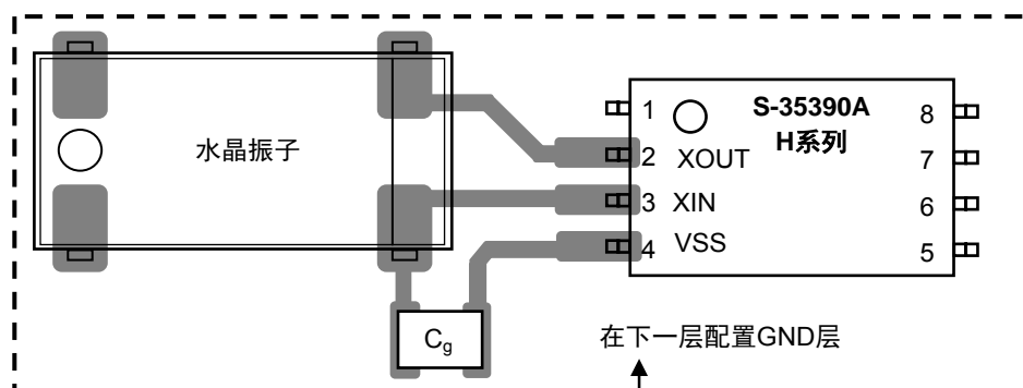
图50 连接图2
